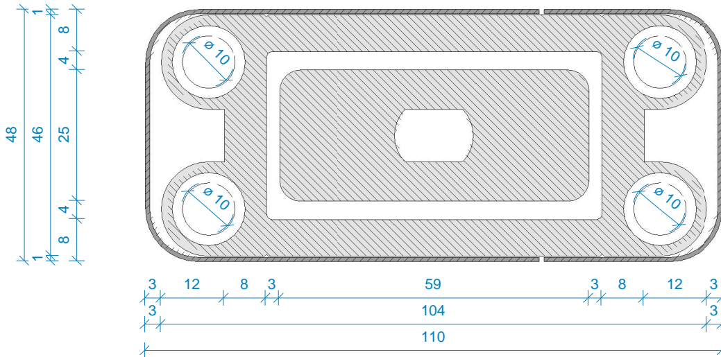
bovenaanzicht 1 : 1
