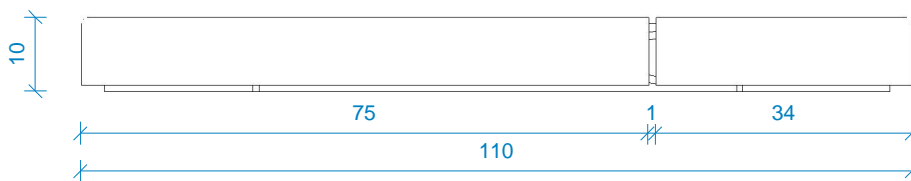
vooraanzicht 1 : 1
