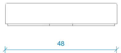
linker zijaanzicht 1 : 1
