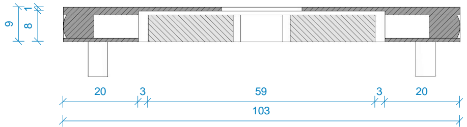
doorsnede 1 : 1
