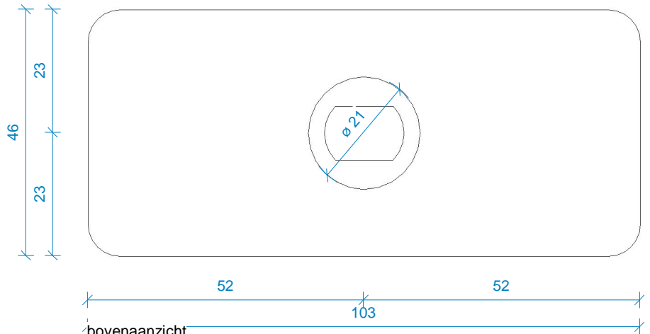
bovenaanzicht 1 : 1
