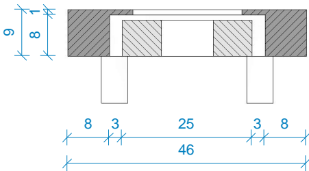
doorsnede 1 : 1
