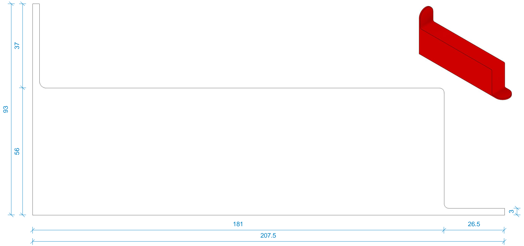
vooraanzicht 1 : 1
