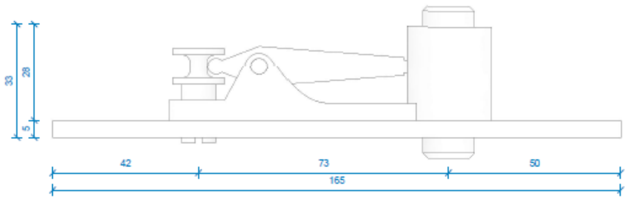
vooraanzicht 1:1
