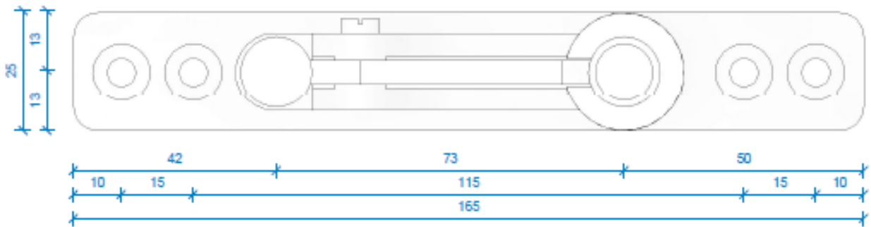
bovenaanzicht 1:1
