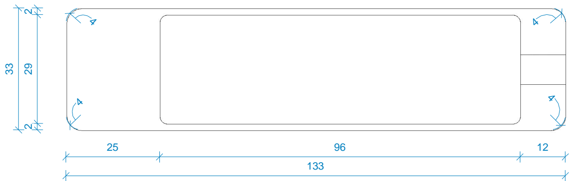
bovenaanzicht 1 : 1
