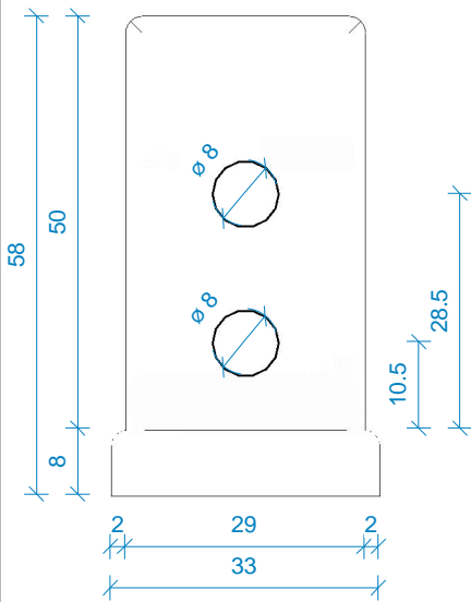
zijaanzicht 1 : 1
