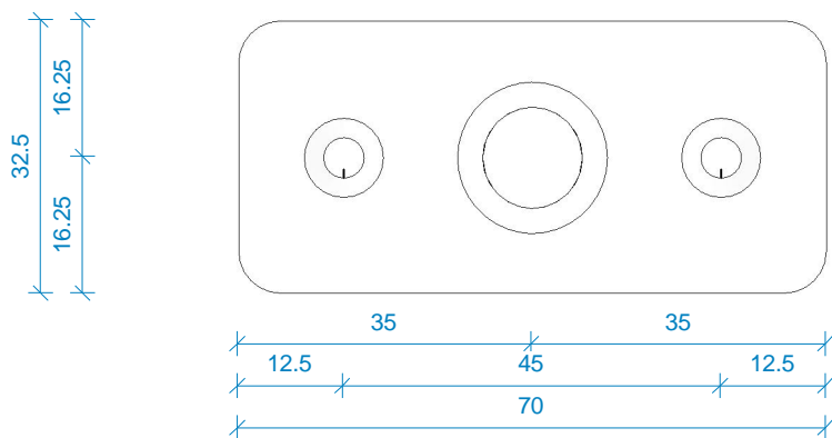
bovenaanzicht (onderplaat) 1 : 1
