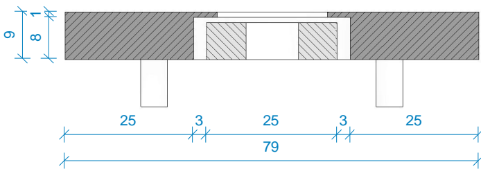
doorsnede 1 : 1
