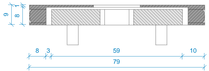
doorsnede 1 : 1
