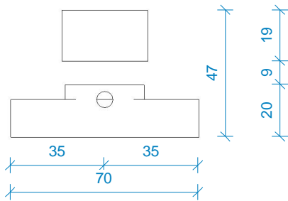
linker zijaanzicht 1 : 2
