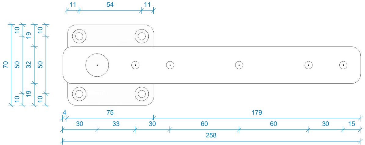
bovenaanzicht 1 : 2
