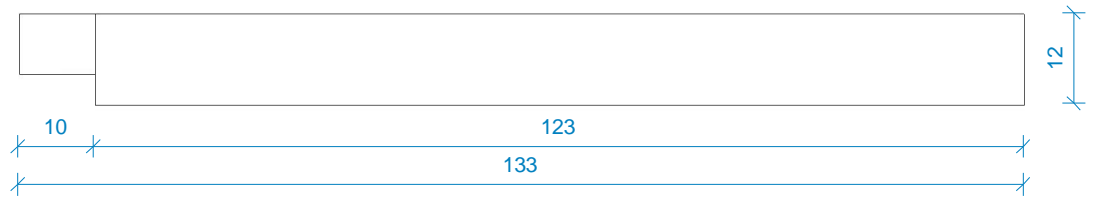
vooraanzicht 1 : 1
