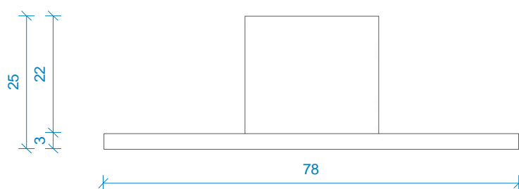
vooraanzicht 1 : 1
