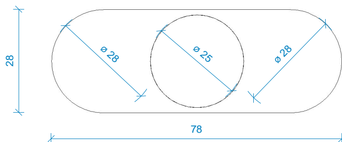
bovenaanzicht 1 : 1
