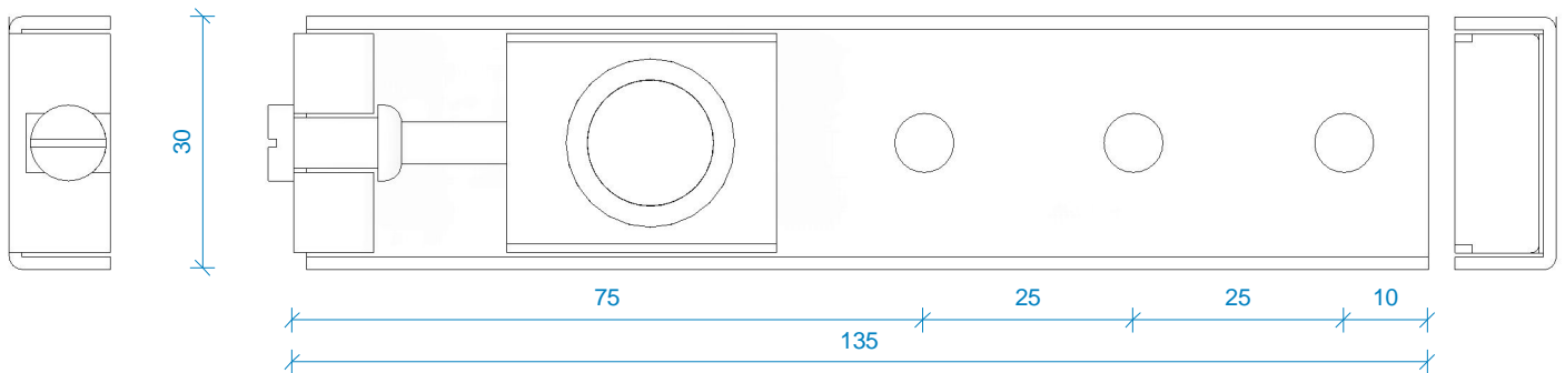
bovenaanzicht 1 : 1
